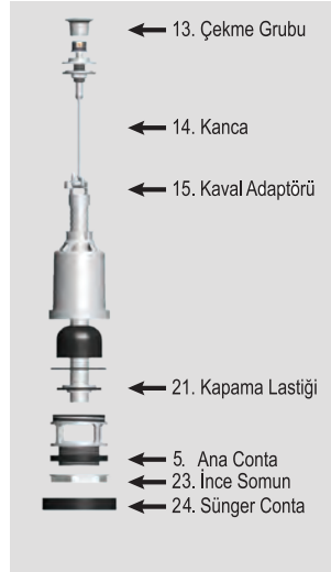
STARMAX İÇ TAKIM 12. Boşaltma Grubu
