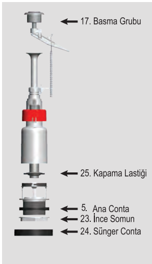
ASSOS İÇ TAKIM 16. Boşaltma Grubu
